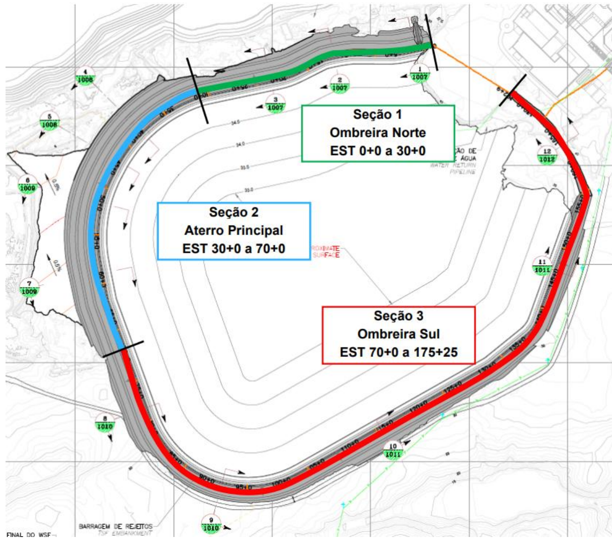
Figura 01 Barragem do Vené I
