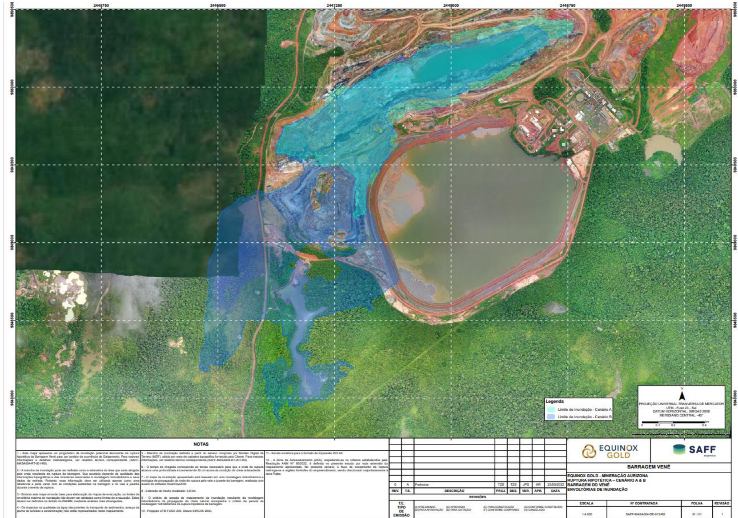
Figura 04 Envoltórias de Inundação – Barragem do Vené I – Cenários A e B
