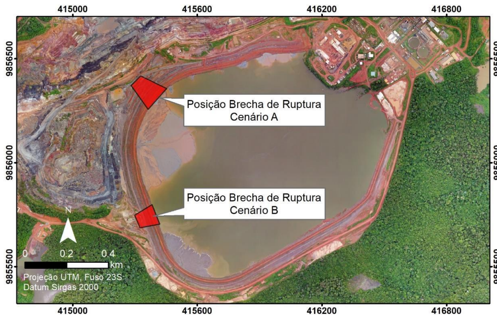
Figura 03 Representação Esquemática da posição da Brecha para simulação de Ruptura Hipotética da Barragem do Vené I para os Cenários A e B.
