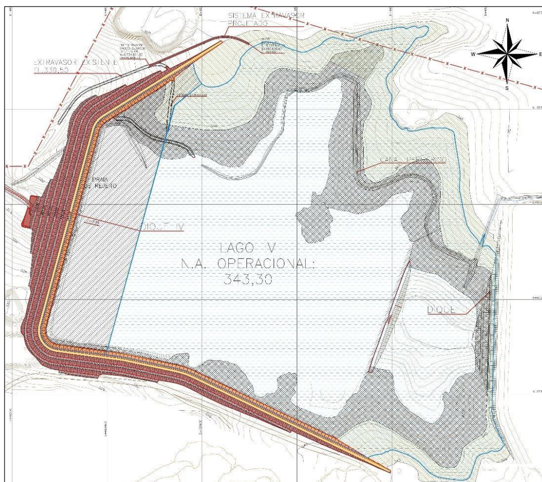
Figura 2 – Vista do arranjo geral do Lago IV – Último alteamento (El. 345,00 m) (Fonte: Fontes Geotécnica, 2020)
