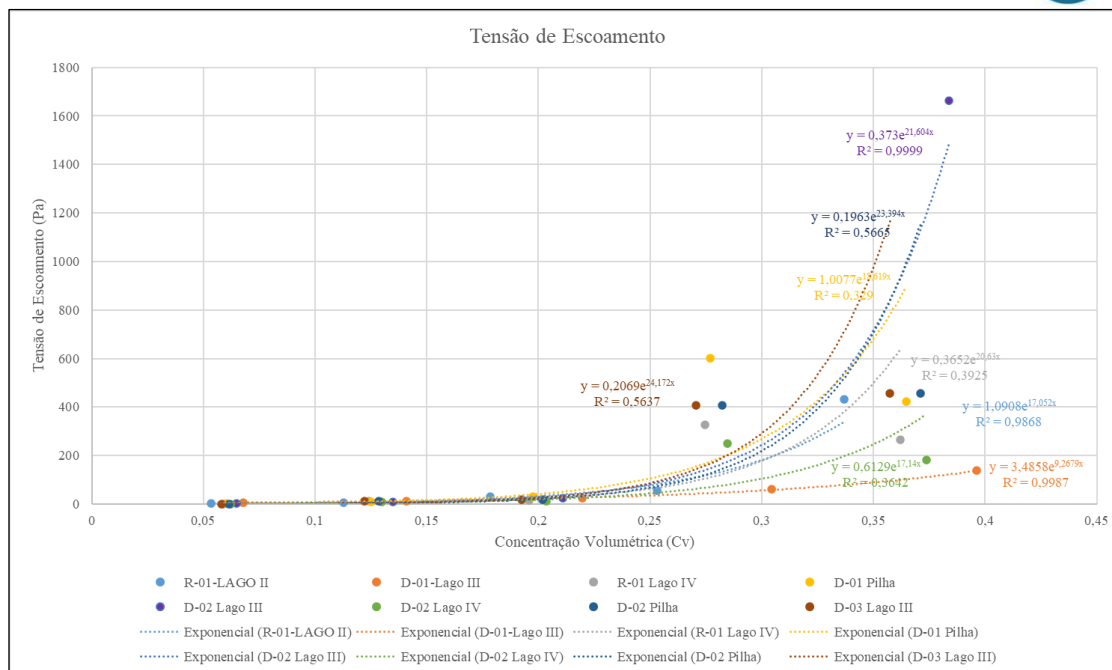
Figura 14 – Reograma de tensão de escoamento das amostras ensaiadas para o Sistema de Disposição de Rejeitos da FBDM
