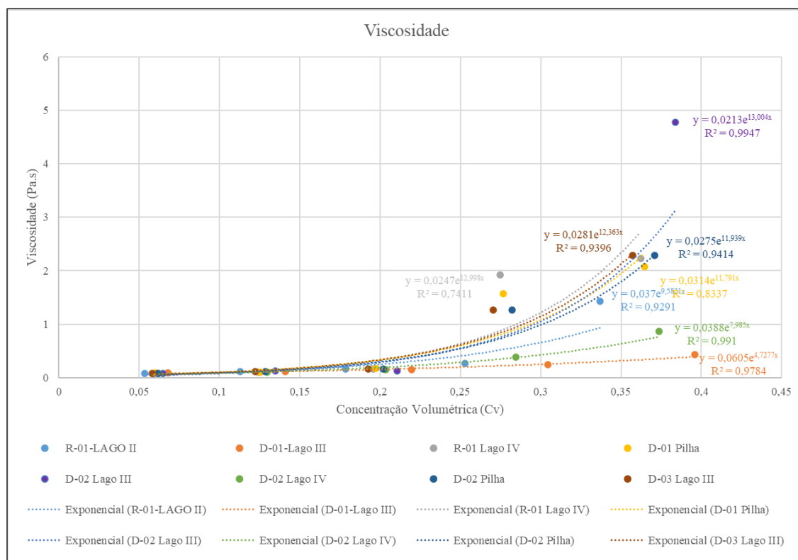
Figura 13 – Reograma de viscosidade das amostras ensaiadas para o Sistema de Disposição de Rejeitos FBDM
